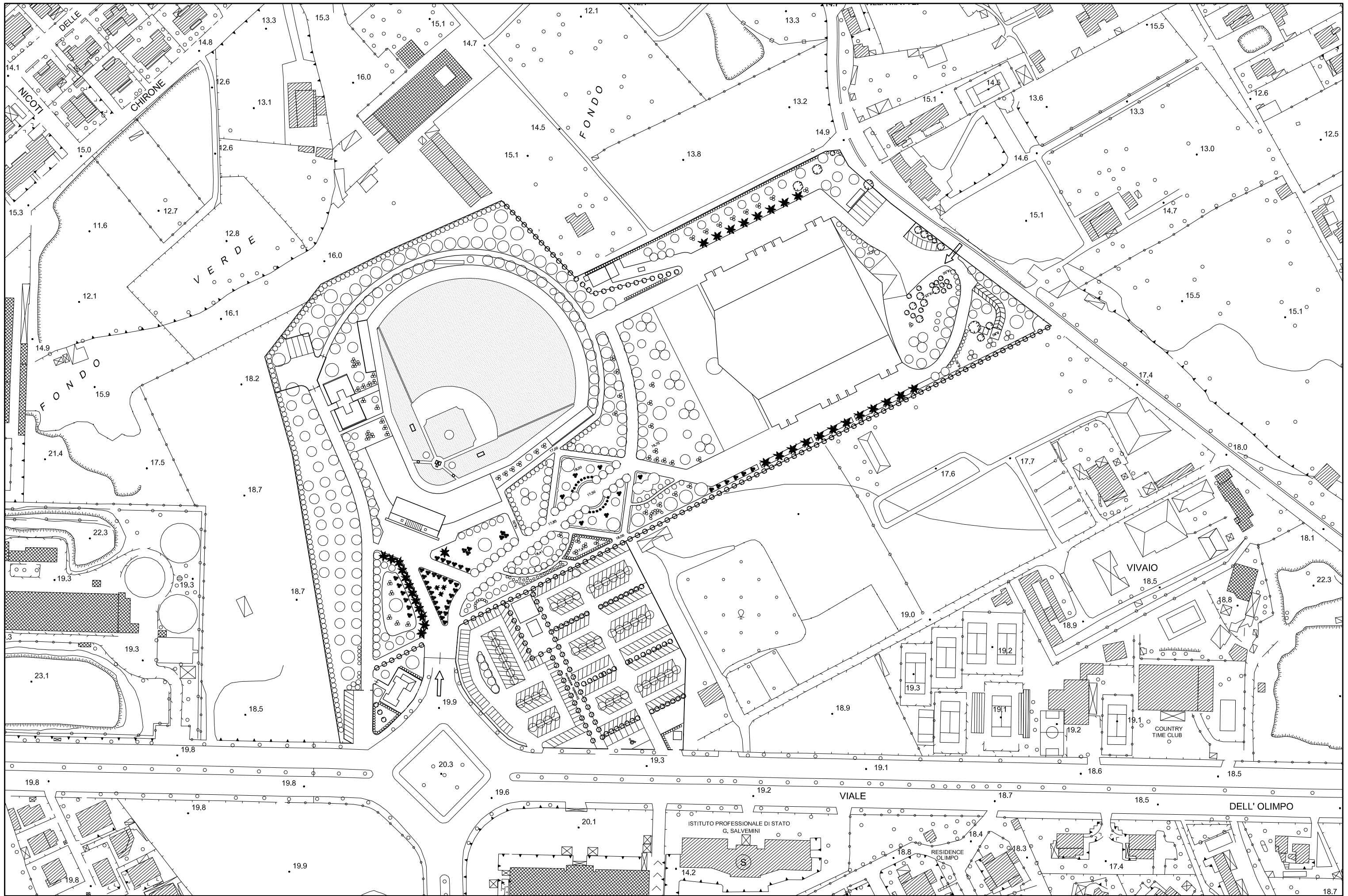
COMUNE DI PALERMO - Aree periferiche da sottoporre ad interventi di riqualificazione urbana mediante procedura di concorso di idee - Cittadella dello sport a San Filippo Neri (ZEN) 2. Planimetria scala 1: 500
